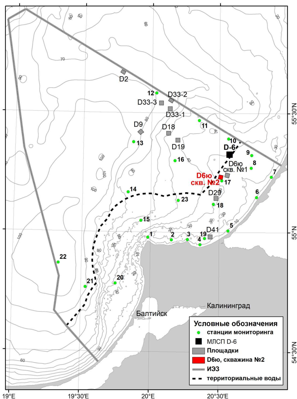
Рисунок 1.1 – Ситуационный план района строительства
